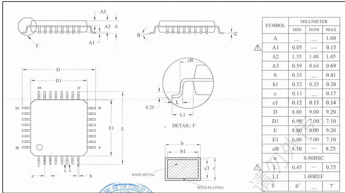
图 4- LQFP32 封装 POD 图
