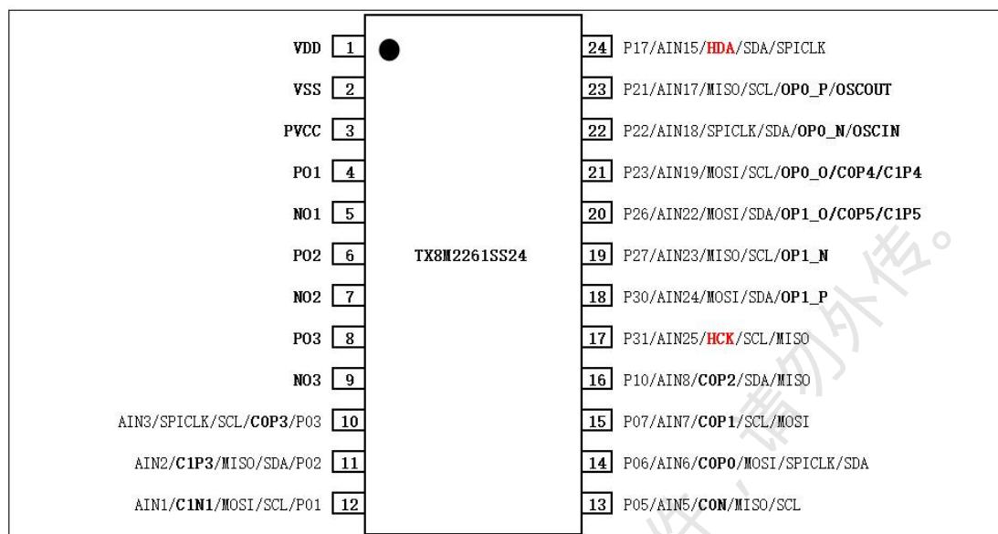
图 1 - TX8M2261SS24 (SSOP24) 封装图
