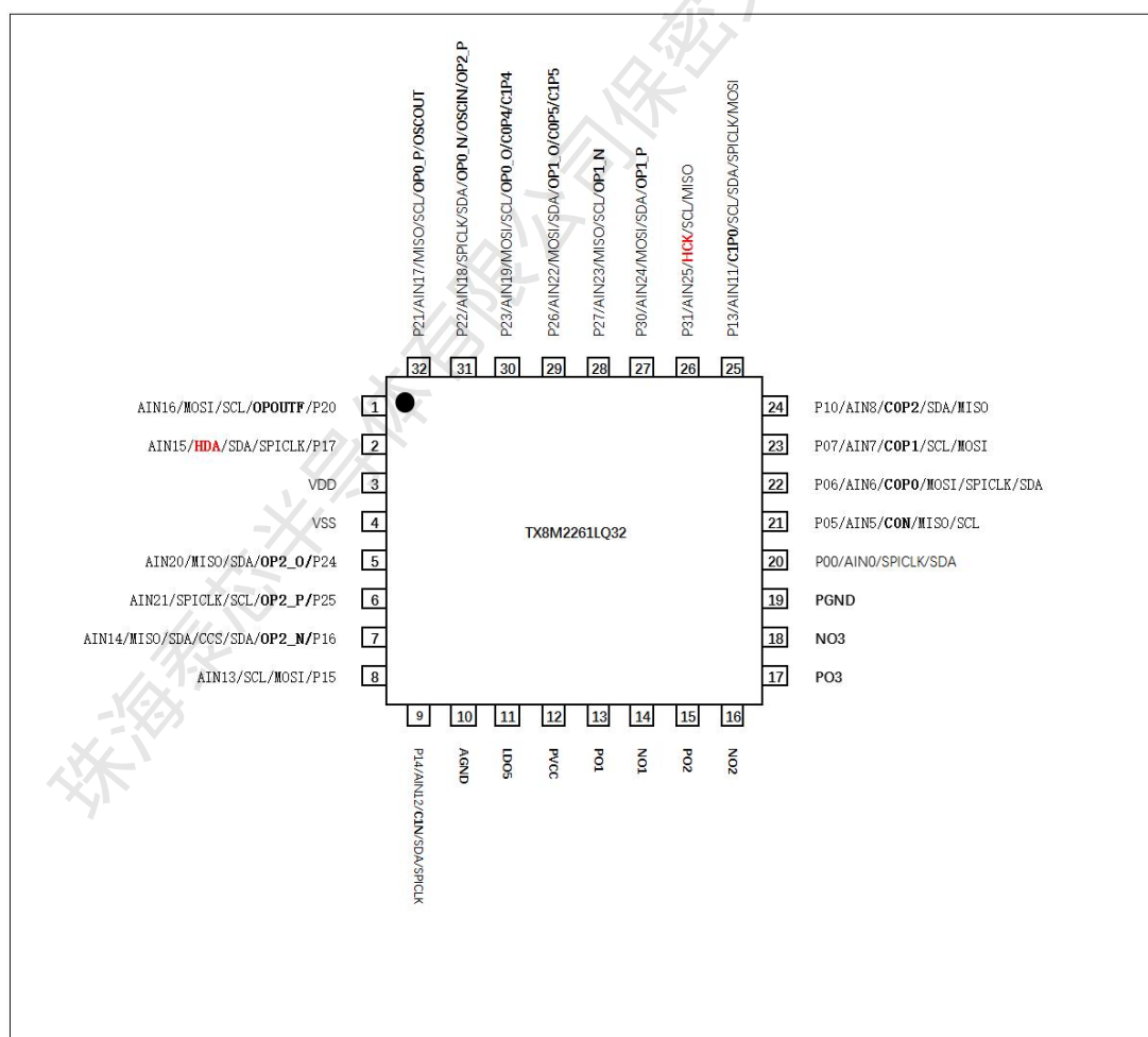
图 2 -TX8M2261LQ32 (LQFP32) 封装图
